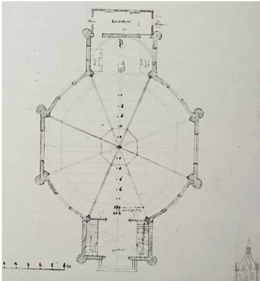
Afb. 2 Grondplan- en kleine opstandtekening van en aantekeningen voor een voorontwerp voor de Hervormde kerk te Helmond, waarschijnlijk uit mei 1847. In het uitgevoerde ontwerp is de driezijdige apsis duidelijker zichtbaar. (Collectie RHCE)
